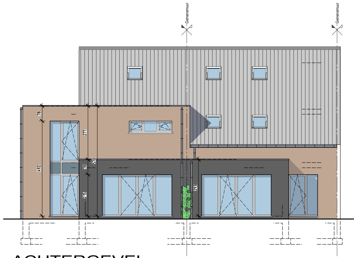
ACHTERGEVEL
